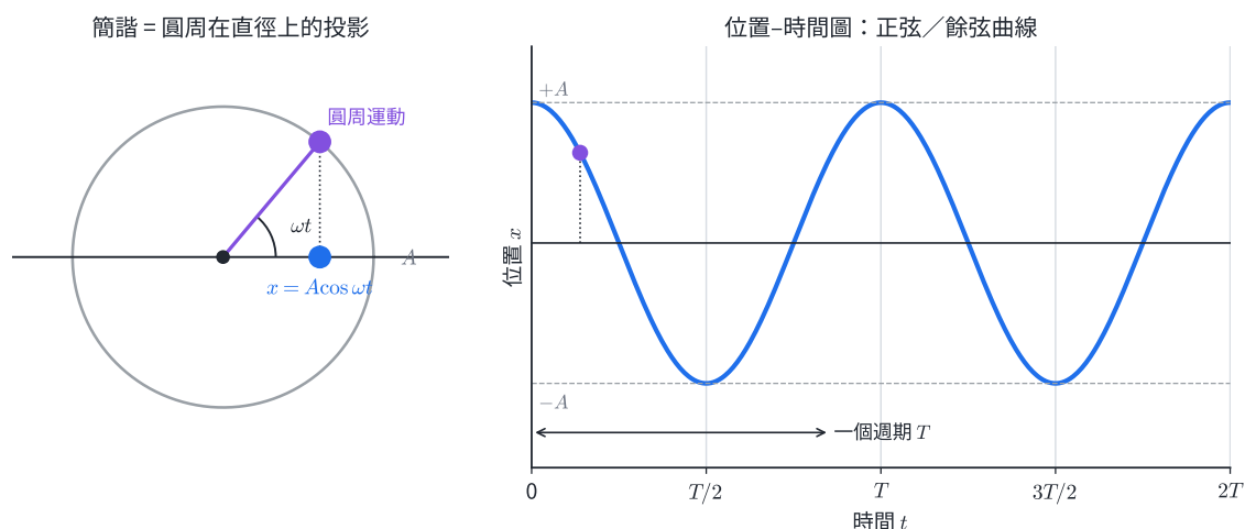
圖 5-3：左——半徑 A 、角速度 \omega 的等速圓周，其在 x 軸上的投影為 x = A \cos \omega t ；右——投影隨時間描出餘弦曲線，一個來回對應圓周轉一圈，週期同為 T = 2\pi/\omega 。
